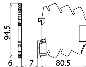
Rozměry DCO SD2 MD 24
