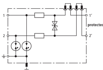
Schéma vnitřního zapojení DCO SD2 MD 24
