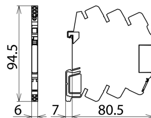
Rozměry DCO SD2 MD 12
