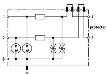
Schéma vnitřního zapojení DCO SD2 ME 24
