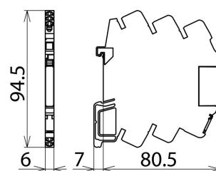
Rozměry DCO SD2 ME 24
