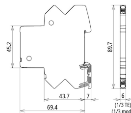
Rozměry BCO CL2 E 48
