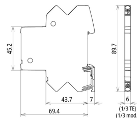
Rozměry BCO CL2 E 24
