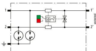
Schéma vnitřního zapojení BCO CL2 BD 48
