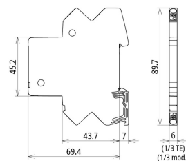
Rozměry BCO CL2 BD 12
