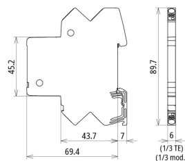
Rozměry BCO CL2 B 180
