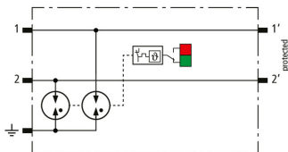
Schéma vnitřního zapojení BCO CL2 B 180
