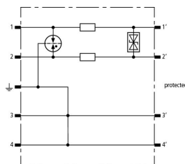
Schéma vnitřního zapojení BSP M2 BD HF 24
