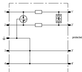
Schéma vnitřního zapojení BSP M2 BD HF 5
