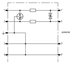
Schéma vnitřního zapojení BSP M2 BD 12
