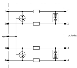
Schéma vnitřního zapojení BSP M4 BD HF 24
