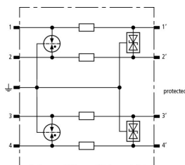
Schéma vnitřního zapojení BSP M4 BE HF 5
