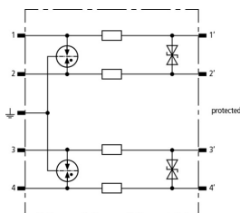
Schéma vnitřního zapojení BSP M4 BD 24
