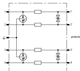
Schéma vnitřního zapojení BSP M4 BD 5
