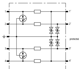
Schéma vnitřního zapojení BSP M4 BE 24
