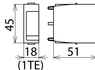
Rozměry DG MOD PV 600
