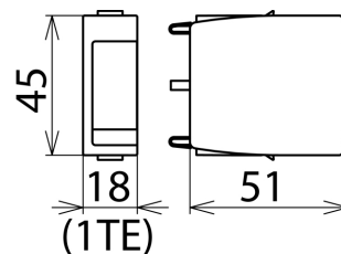
Rozměry DG MOD PV SCI 600
