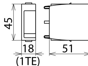
Rozměry DG MOD 75 VA
