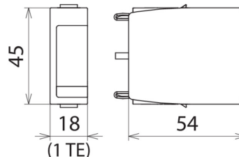
Rozměry DG MOD H A NPE
