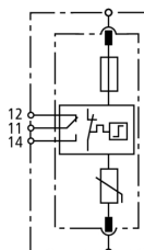
Schéma vnitřního zapojení DG MOD E CI WE 440
