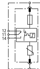
Schéma vnitřního zapojení DG MOD E CI 440
