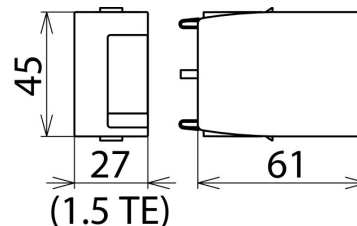
Rozměry DG MOD E CI 440
