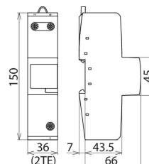
Rozměry DGPM 440
