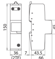
Rozměry DGPM 1 255
