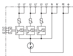
Schéma zapojení DCU EMOB 2 32
