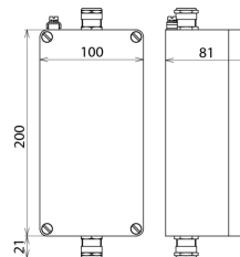
Rozměry ALGA 5
