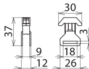
Rozměry AK 35 SN 18X3 GG
