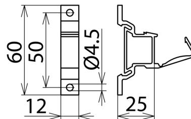
Rozměry SH 18X3 K
