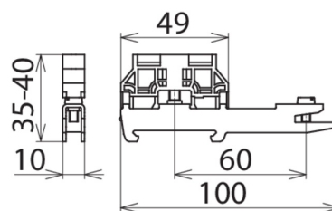
Rozměry SH1 18X3 ST
