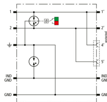
Schéma vnitřního zapojení DBX TC B 180
