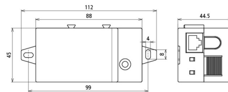
Rozměry DBX TC B 180
