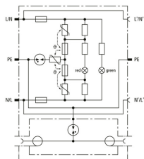
Schéma vnitřního zapojení DPRO 230 TV
