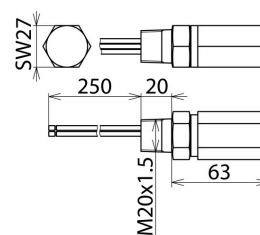
Rozměry DPI CD EXD 230 24 M
