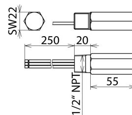
Rozměry DPI CD EXD 24 N
