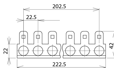
Rozměry MB2 10 LSA
