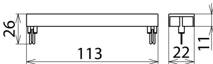
Rozměry EF 10 DRL
