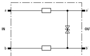
Schéma vnitřního zapojení DRL RD 60
