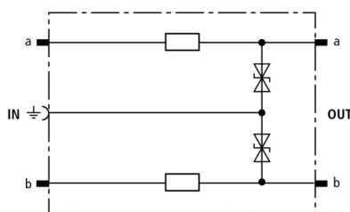
Schéma vnitřního zapojení DRL RE 180
