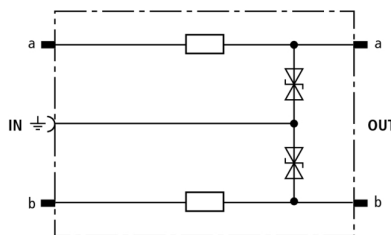
Schéma vnitřního zapojení DRL RE 48
