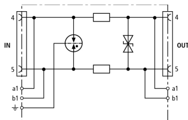
Schéma vnitřního zapojení BVT TC
