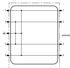
Schéma vnitřního zapojení BXT M4 E
