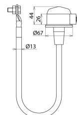
Rozměry EXFS L100
