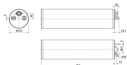
Rozměry DASD 45 LP 100 T
