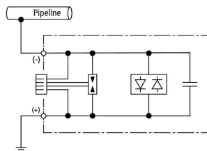
Schéma vnitřního zapojení DASD 45 LP 100 T
