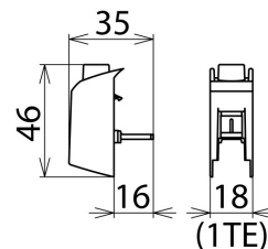
Rozměry STAK 25
