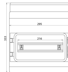
Rozměry IGA 12 IP65
