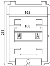
Rozměry IGA 6 IP54
