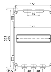
Rozměry IGA 7 IP54
