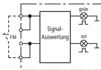
Schéma vnitřního zapojení DPAN L
