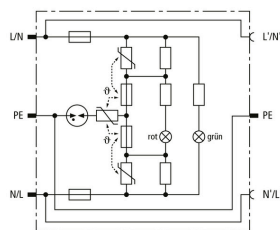
Schéma vnitřního zapojení DPRO 230
