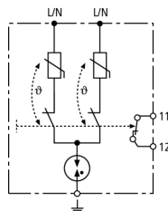
Schéma vnitřního zapojení VC 280 2
