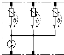
Schéma vnitřního zapojení DR MOD 4P 255
